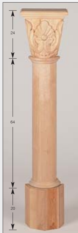
Half-column / Halbsäule / Demi-Balustre / Halve zuil Art.Nr. 50.1120.024.00 H 108 cm Top B 24, T 12 cm Base B 20, T 10 cm
