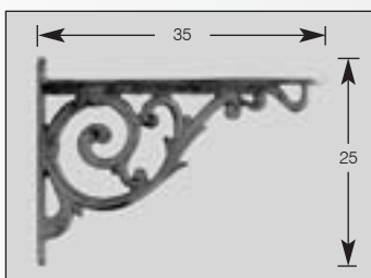
Art.Nr. 72.3020.025.00
