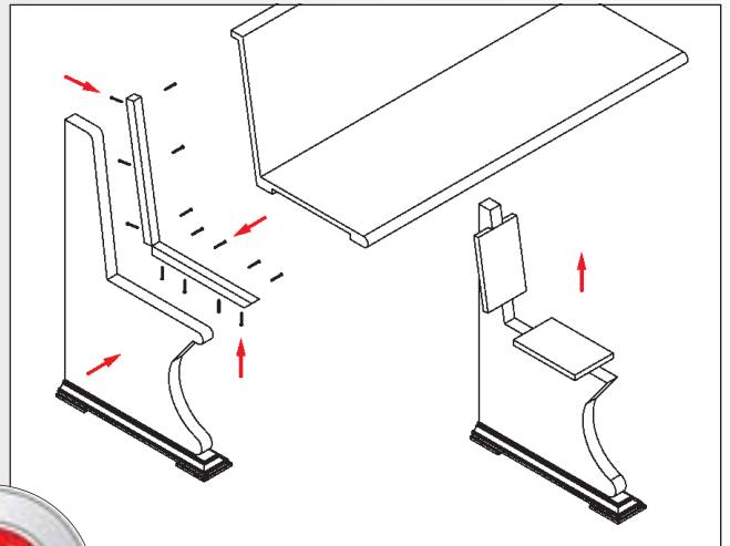
High bench support Unterbau Départ de banc haut Onderstel Art.Nr. 50.7110.076.00 H 111, T 57,5 cm
