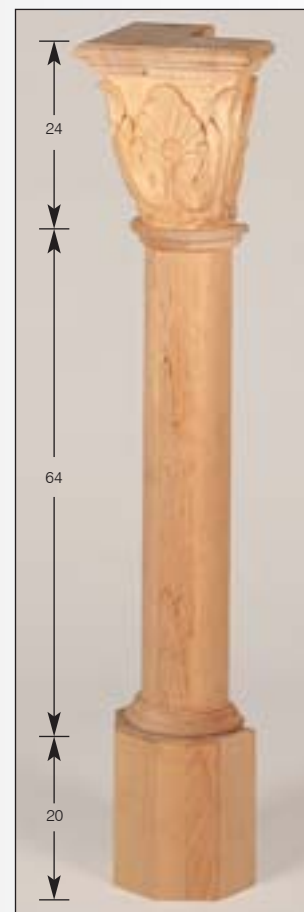
Corner-column 90° / Ecksäule 90° / Balustre 90° / Hoek zuil 90° Art.Nr. 50.1130.024.00 H 108 cm Top 24 x 24 cm Base 20 x 20 cm
