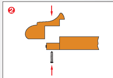
Round external moulding 90° Außen-Rundecke 90° Coin extérieur arrondi 90° 90° buiten ronding Art.Nr. 50.4410.060.00 Ø 60 cm (bar top / Plattenmaß / plateau / bladmaat)
