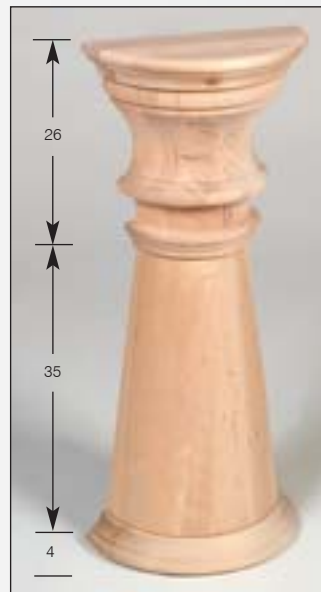
Half-column / Halbsäule / Demi-Balustre / Halve zuil Art.Nr. 50.1050.030.00 H 65 cm Top B 30, T 15 cm Base B 30, T 15 cm
