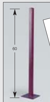
Steel support for heavy baluster (raw) / Innenkern für Antrittsposten (roh) / Fixation au sol (brut) / Stalen flens (onbewerkt) Art.Nr. 50.0490.010.18 for / für / pour / voor 50.0150.012.00, 50.0350.015.00
