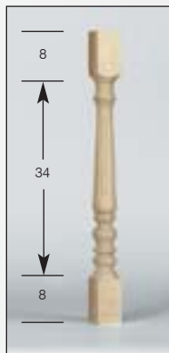
Column / Säule / Balustre / Baluster Art.Nr. 50.0100.004.00 ∅ 4,5 cm
